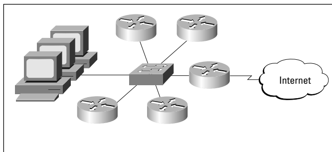
Figura 3: connessione effettuata con topologia a stella
