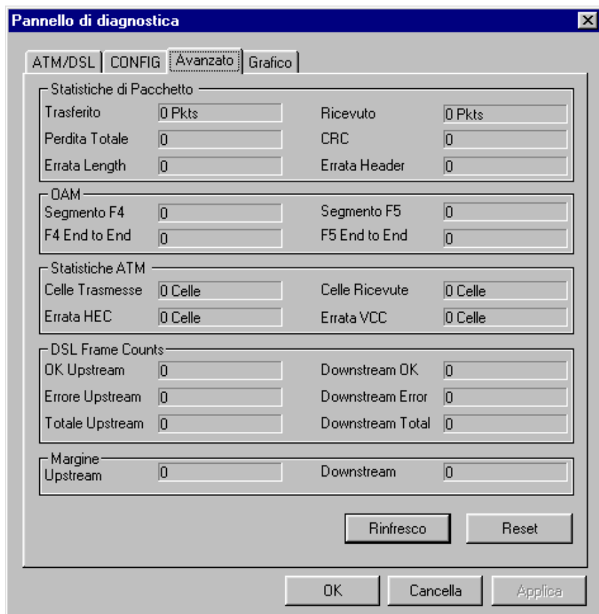
Figura 16: Pannello di diagnostica informazioni avanzate
