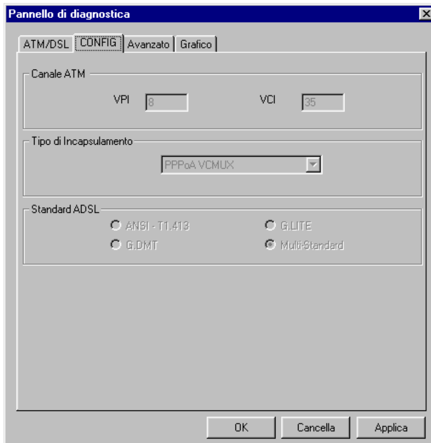
Figura 15: Pannello di diagnostica configurazione linea ADSL
