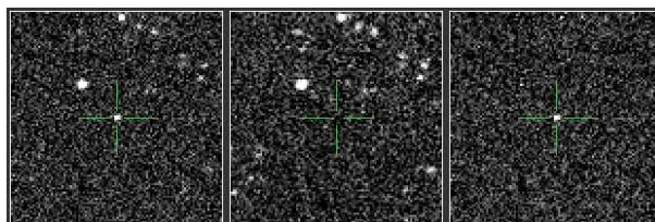
PTF ID: 10vqv - Ia
