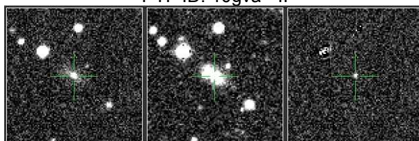
PTF ID: 10mwb - Ia
