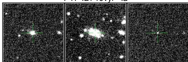
PTF ID: 10wyq - Ia
