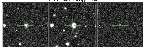
PTF ID: 10xtu - Ia
