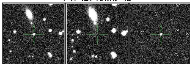
PTF ID: 10xgc - Ia
