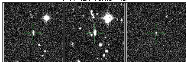
PTF ID: 10yzt - IIa
