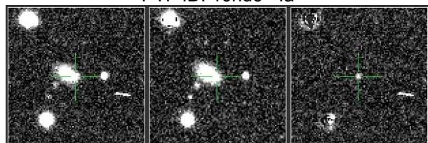
PTF ID: 10urj - Ia
