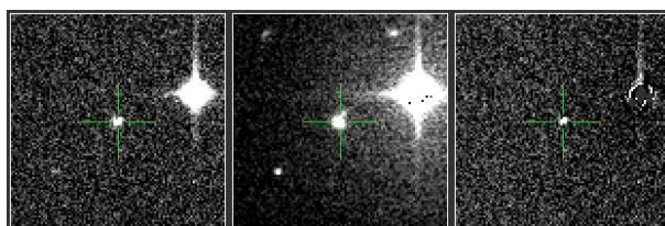
PTF ID: 10wnt - Ia
