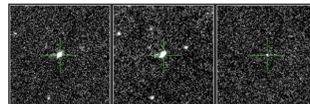
PTF ID: 10xgx - Ia
