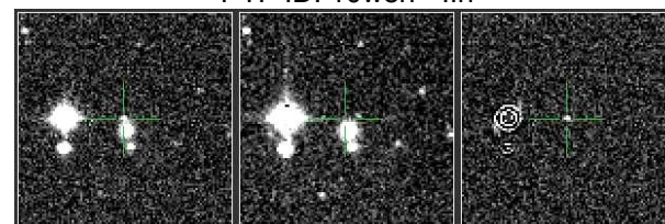
PTF ID: 10xgp - Ia
