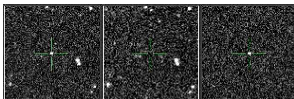
PTF ID: 10ops - Ia pec
