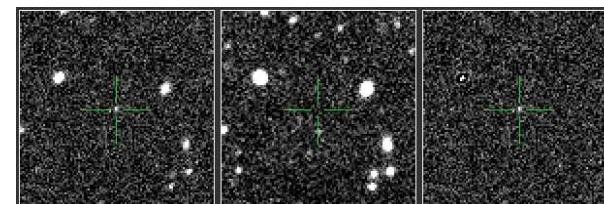
PTF ID: 10guz - Ia pec
