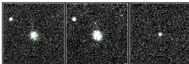
PTF ID: 10gva - II
