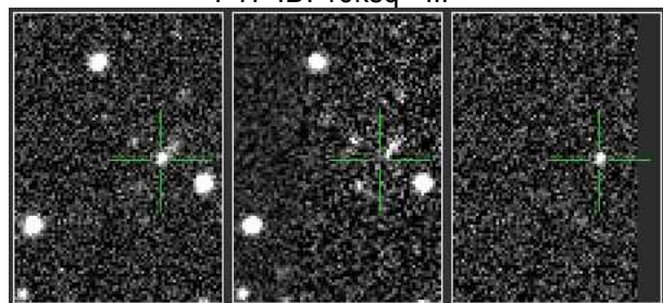
PTF ID: 10ndc - Ia
