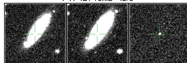
PTF ID: 10ygu - Ia pec
