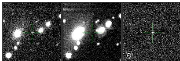
PTF11rmu - Ia
