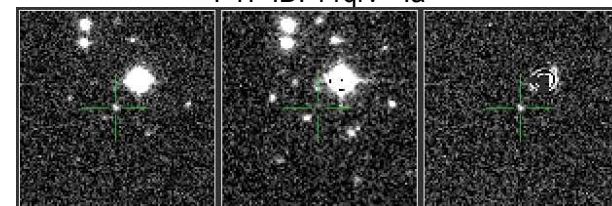
PTF11mq - Ia
