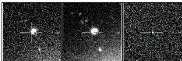
PTF11rpz - Ia
