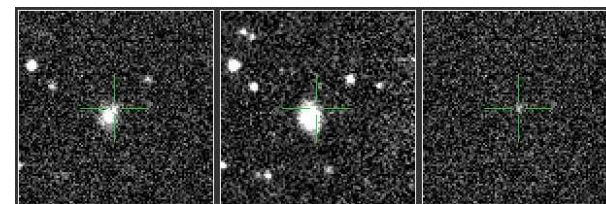
PTF11rrq - Ia
