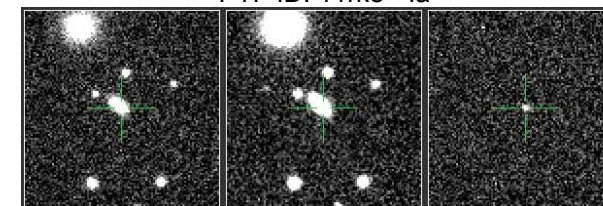
PTF11rpj - Ia
