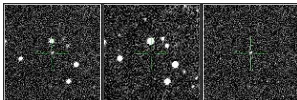
PTF12gmq - la
