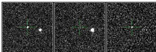
PTF12dyv - Ia
