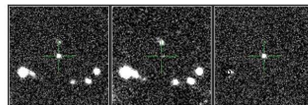
PTF12box - Ia
