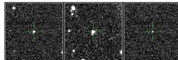
PTF12dcg - Ia
