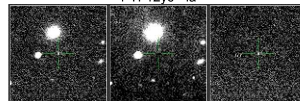
PTF12ass - la
