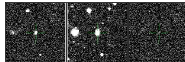
PTF12eac - Ia
