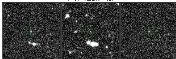
PTF12vr - la
