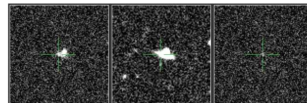
PTF12cni - Ia
