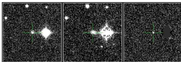
PTF12glz - IIIn
