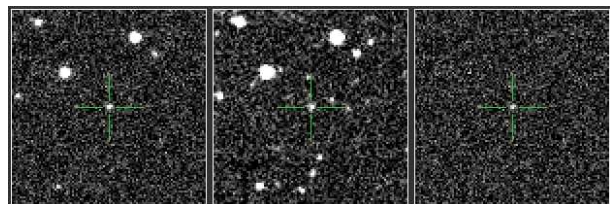
PTF12dem - Ia
