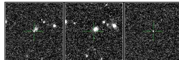
PTF12gmu - la
