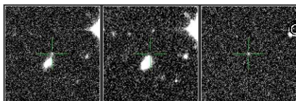
PTF12ast - Ia
