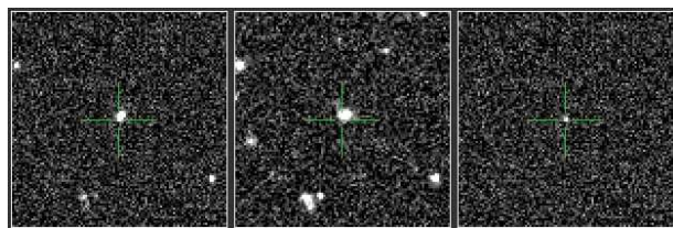
PTF12dst - Ia
