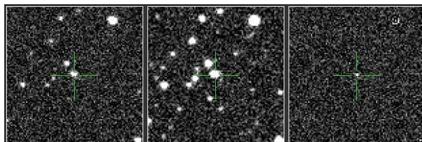
PTF12brj - Ia
