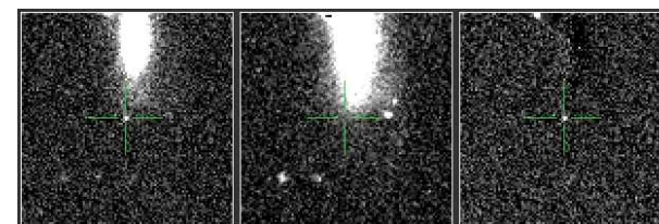
PTF12bok - la
