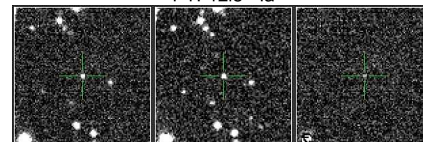
PTF12yc - la
