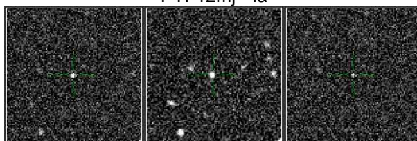
PTF12ax - la
