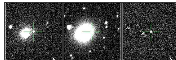
PTF12dxm - Ia
