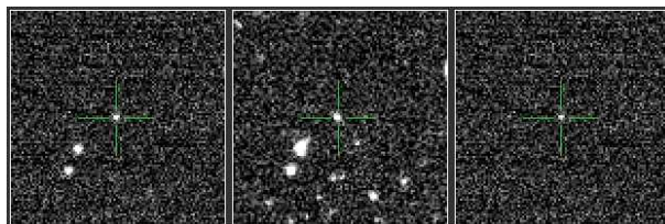
PTF12eab - Ia
