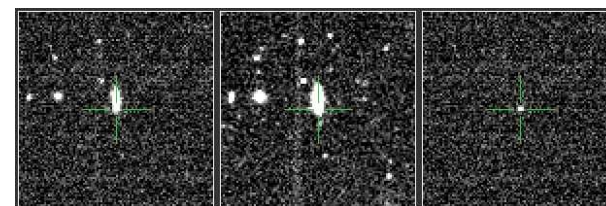
PTF12ccy - Ia
