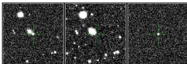
PTF12ccx - Ia
