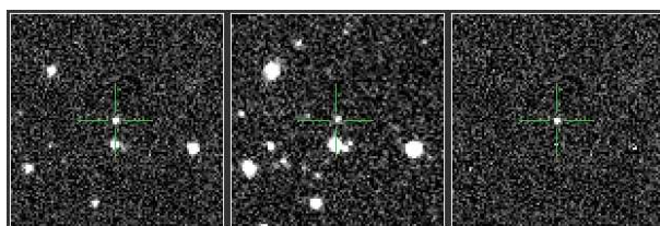
PTF12bod - Ia
