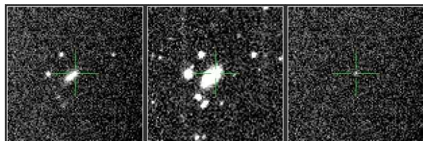
PTF12gkn - la
