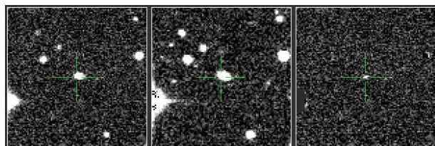
PTF12dyr - Ia
