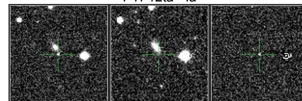
PTF12ie - la
