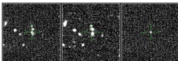
PTF12asw - Ia
