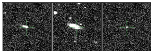
PTF12gmv - la
