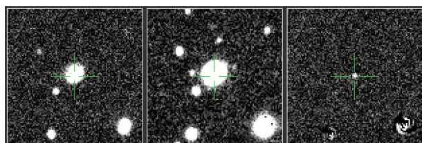
PTF12bmr - Ia
