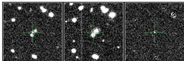
PTF12bpy - II
