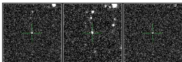
PTF12elj - la
