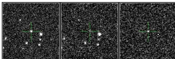
PTF12czu - Ia
