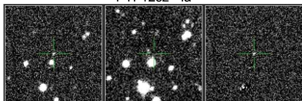
PTF12zg - la
