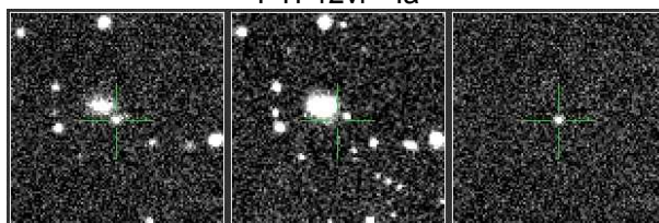
PTF12art - la
