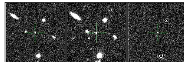
PTF12cdq - Ia
