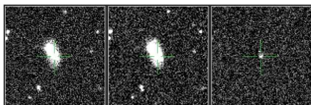
PTF12ggb - la
