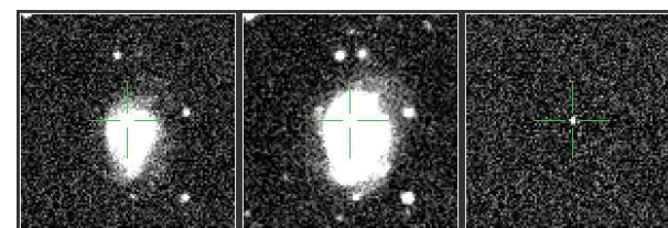
PTF12giy - la
