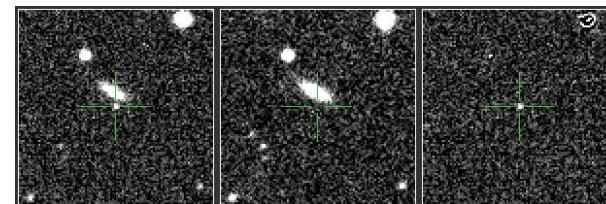
PTF12btr - Ia
