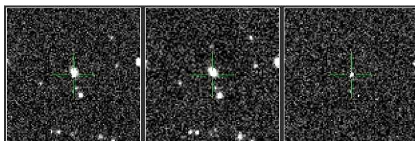
PTF12gmy - la
