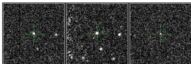
PTF12bvz - Ia
