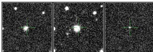
PTF12mj - la
