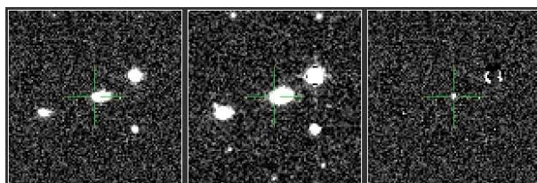
PTF12cdb - Ia
