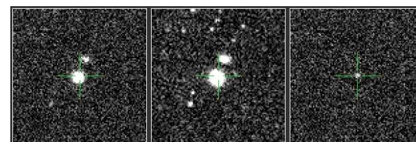
PTF12eut - la
