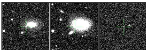
PTF12ghy - la
