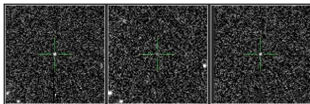
PTF12ejf - Ia
