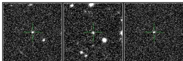
PTF12lz - la
