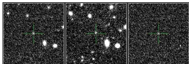
PTF12cyd - Ia
