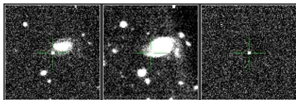
PTF12dco - Ia
