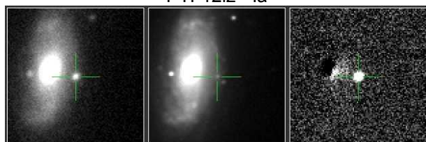
PTF12os - lib
