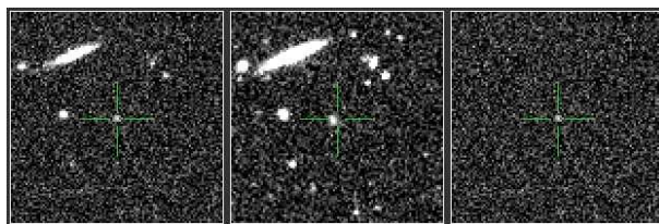
PTF12ejg - Ia
