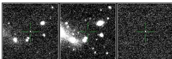
PTF12etn - la
