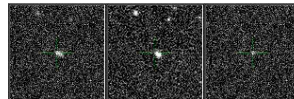
PTF12ta - la
