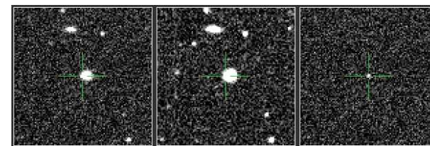
PTF12elc - Ia
